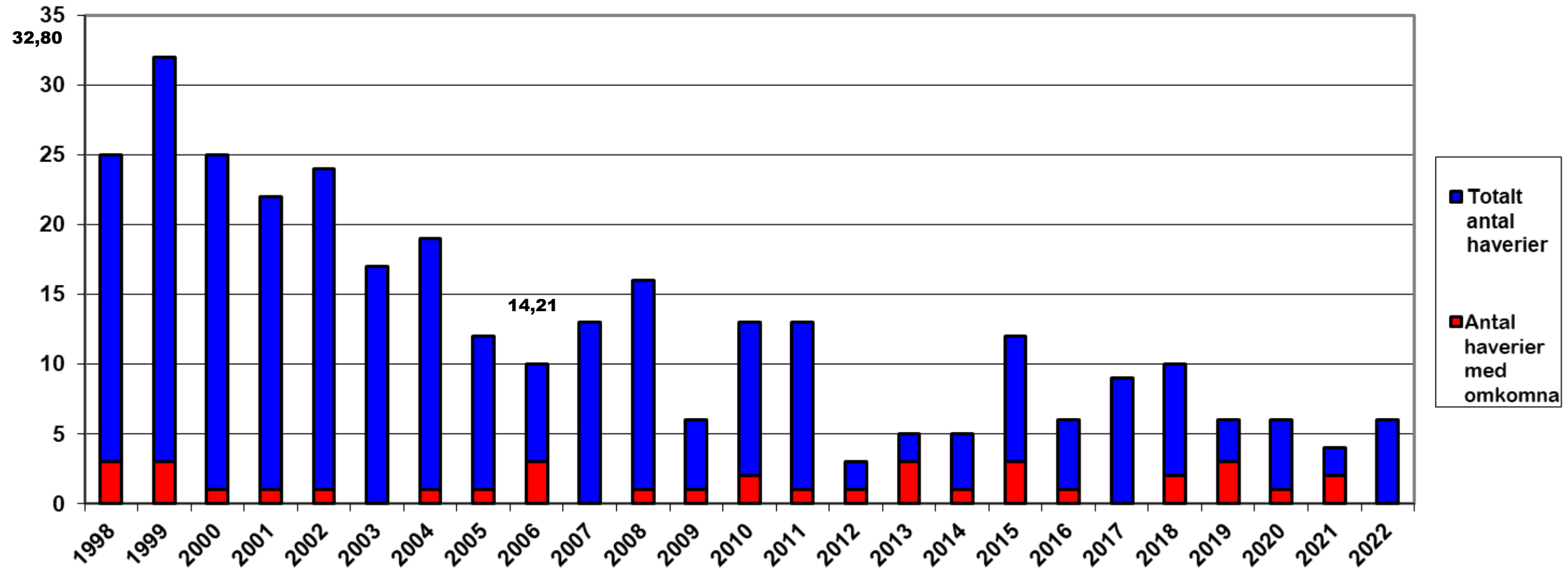
Haverier med normal och X-klassade privatflygplan Ej UL och ej skolflygning Kurvan visar frekvensen per 100.000 flygtimmarr
